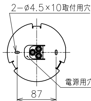
取付板詳細 S:1/5
